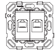
insert RJ45 UTP 0403-03 Cat5e 0403-13 Cat6
